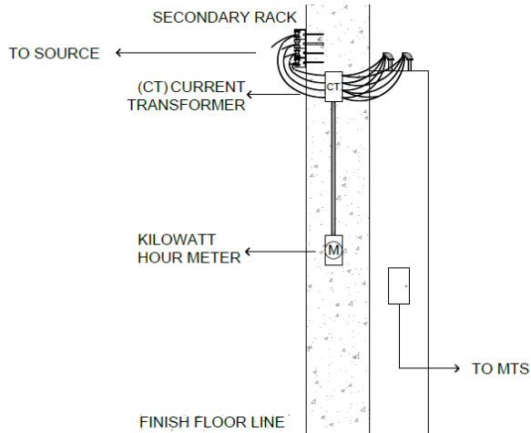
6 E-1 S E C O N D A R Y R A C K A N D S E R V I C E E N T R A N C E D E T A I L N O T T O S C A L E
