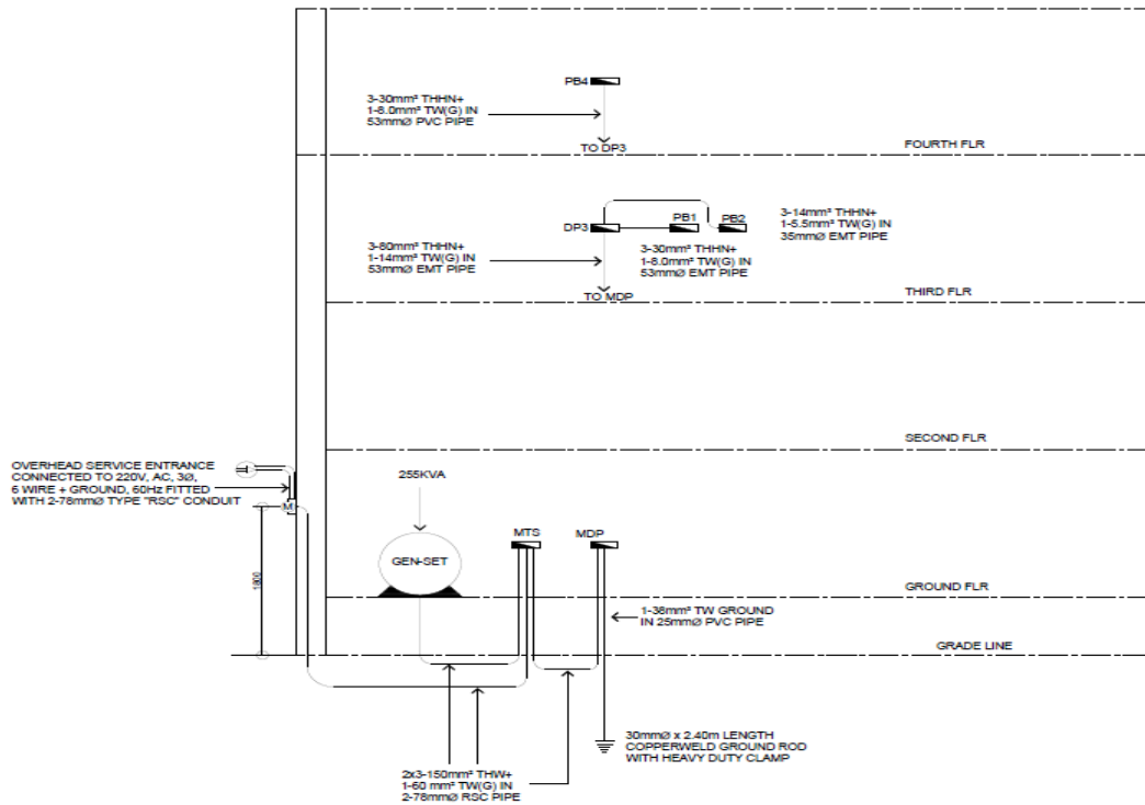
1 R I S E R D I A G R A M E-3 N O T T O S C A L E
