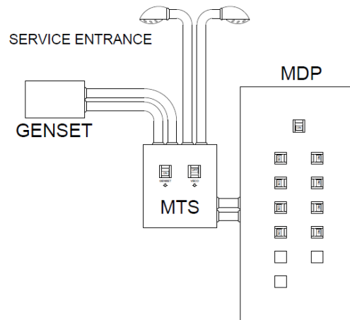
1 E-2 S E R V I C E E N T R A N C E A N D P A N E L B O A R D S D E T A I L N O T T O S C A L E
